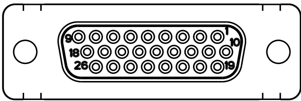
SIZE 2 SCALE 2:1
