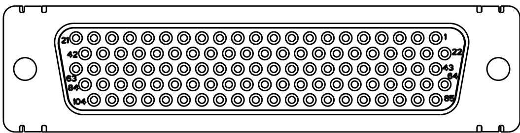
SIZE 6 SCALE 2:1
