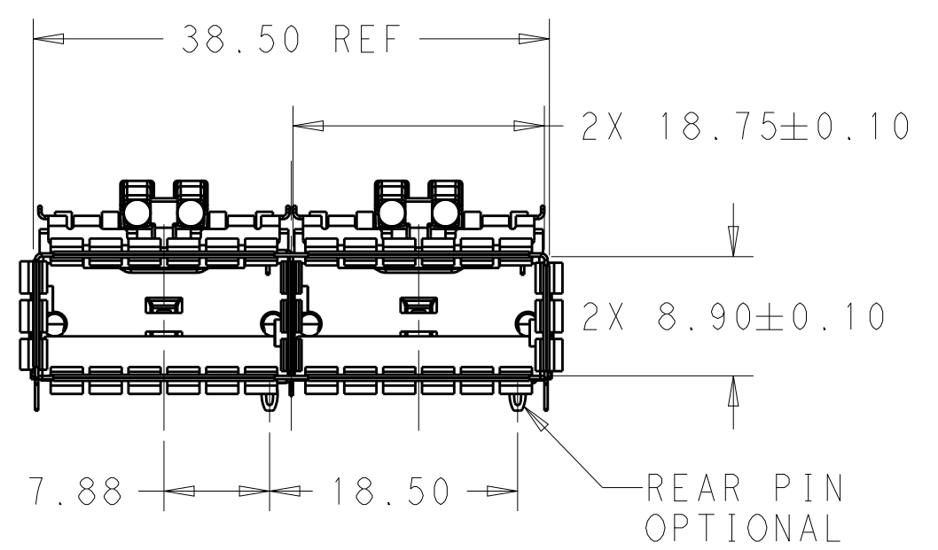
SCALE 2:1
