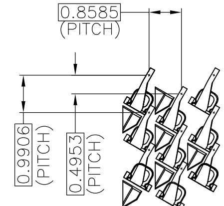
DETAIL P(10:1)
