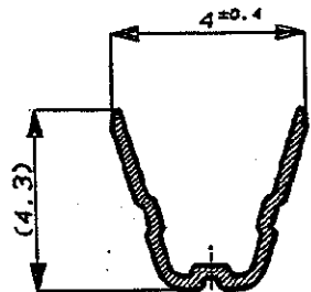
断面 D-D SECT. D-D
