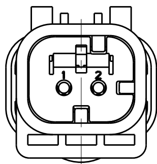
1717672-2 SCALE 2:1
