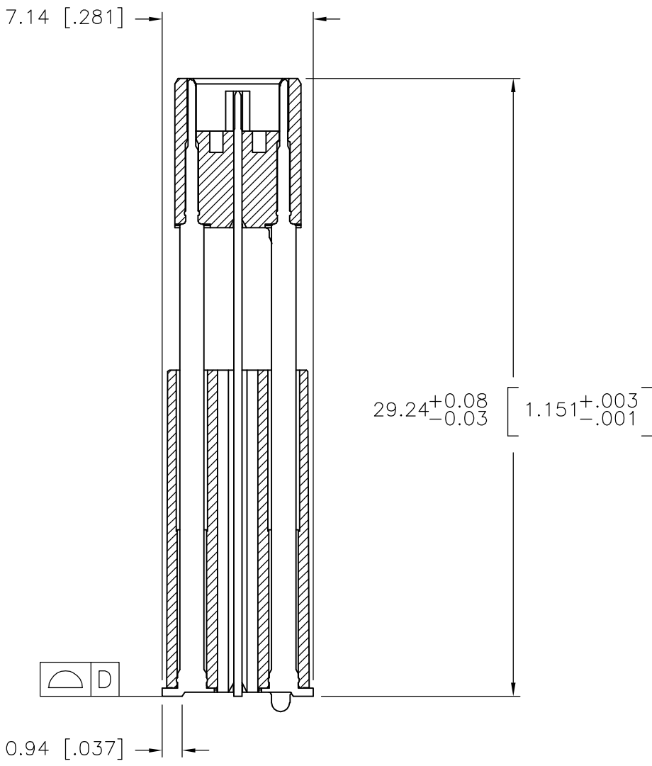
SECTION A-A
