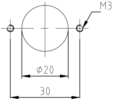
Panel cut-out nur für PN 7-2
