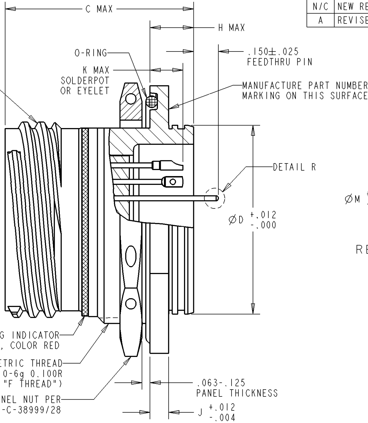
SECTION A-A
