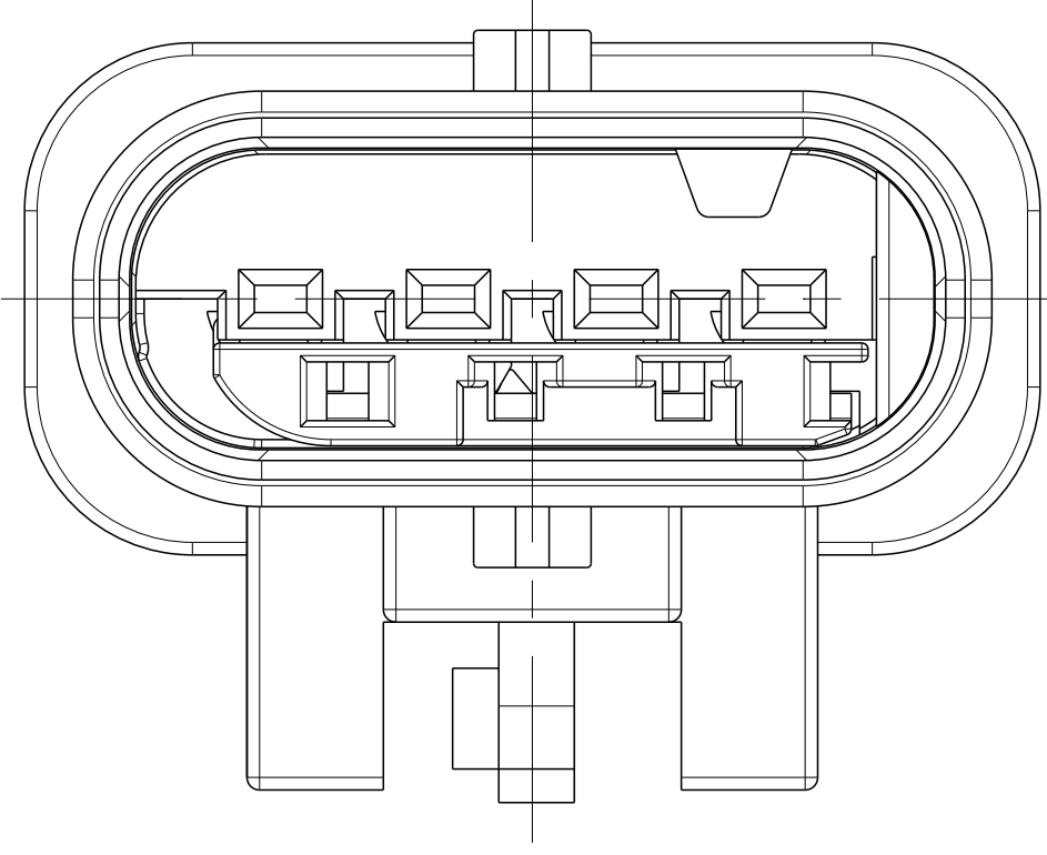
RETAINER MOVING DIRECTION 2. Kontaktsicherung Verschiebeweg
