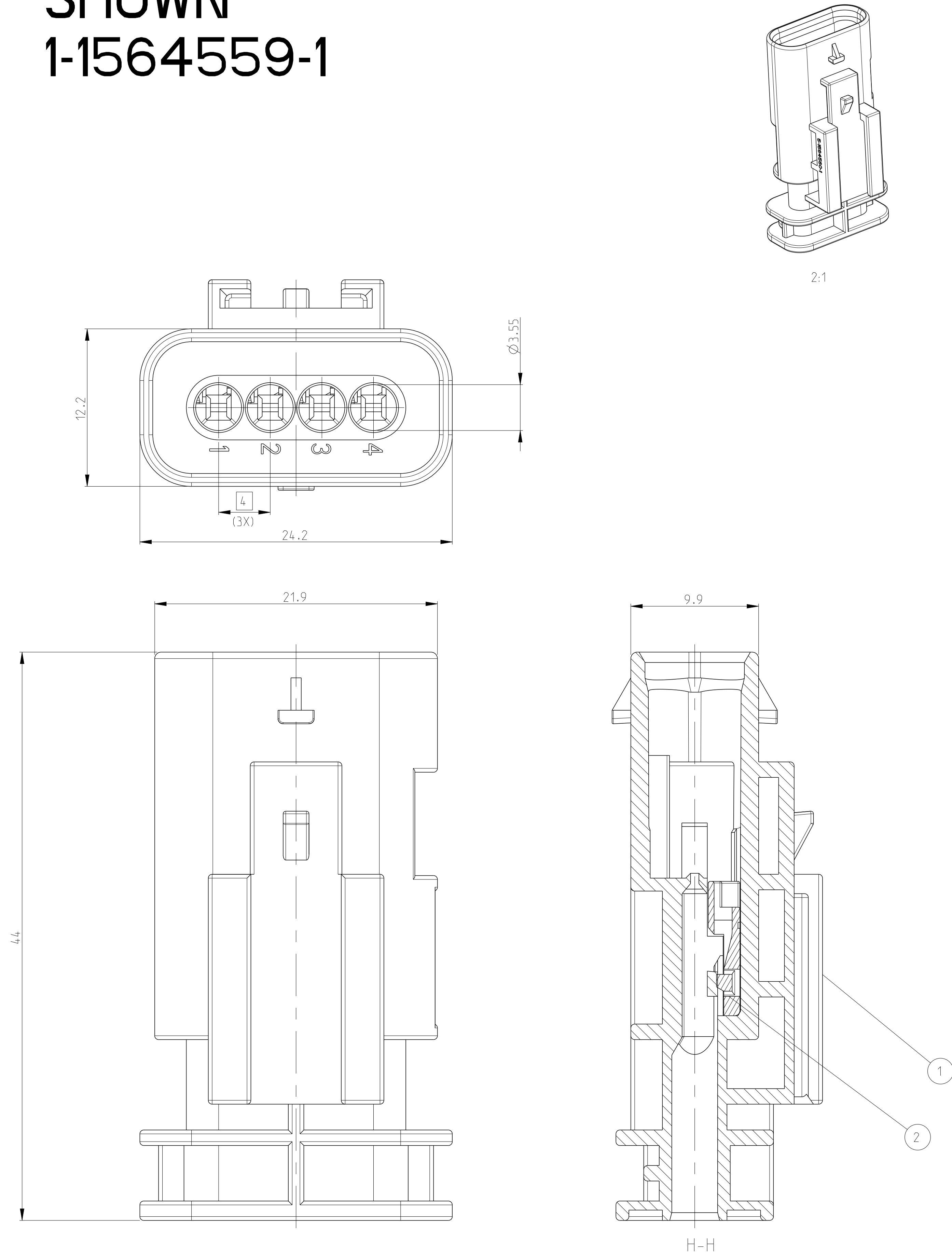
RETAINER IN PRE LOCKED POSITION Kontaktsicherung in Vorraststellung
