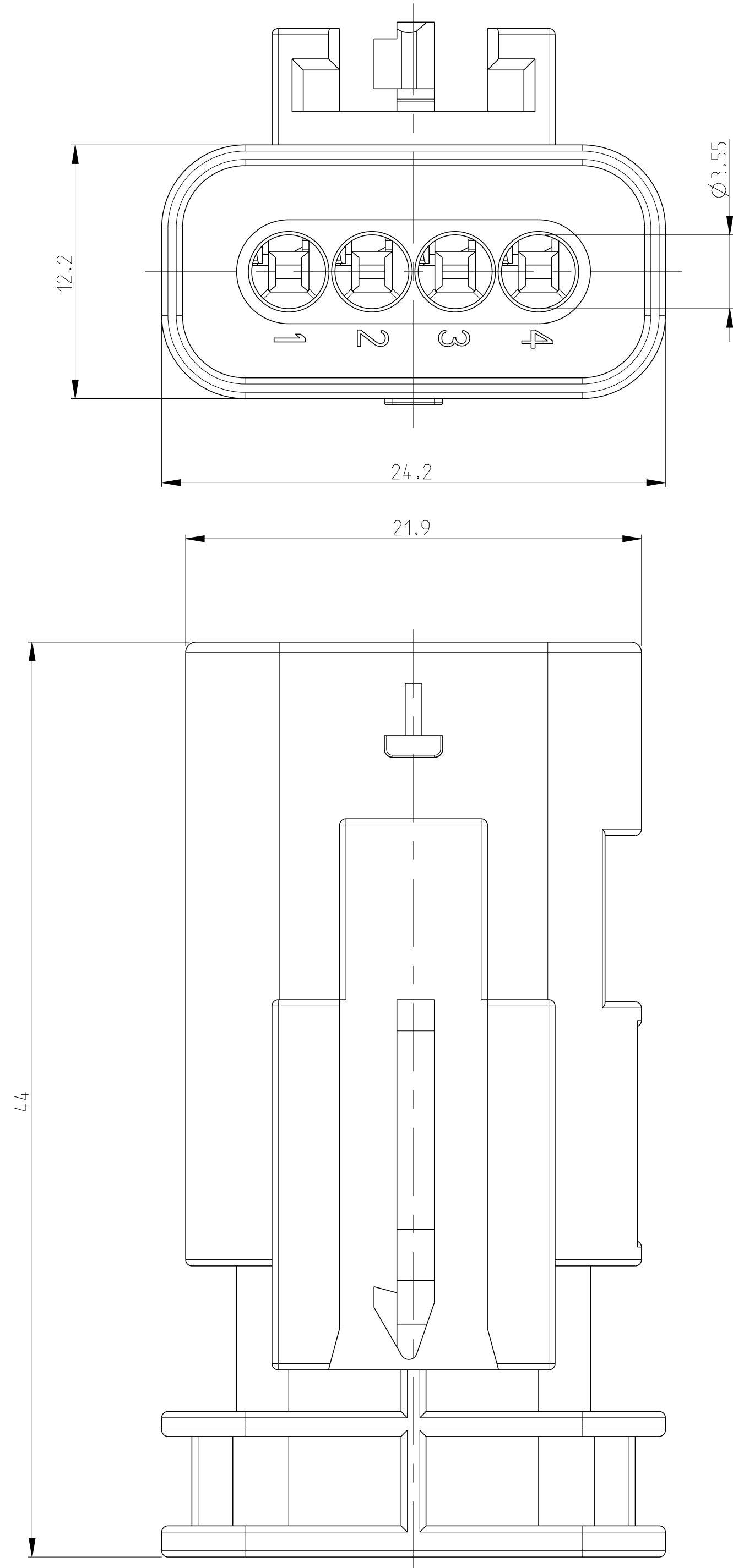
RETAINER IN PRE LOCKED POSITION Kontaktsicherung in Vorraststellung
