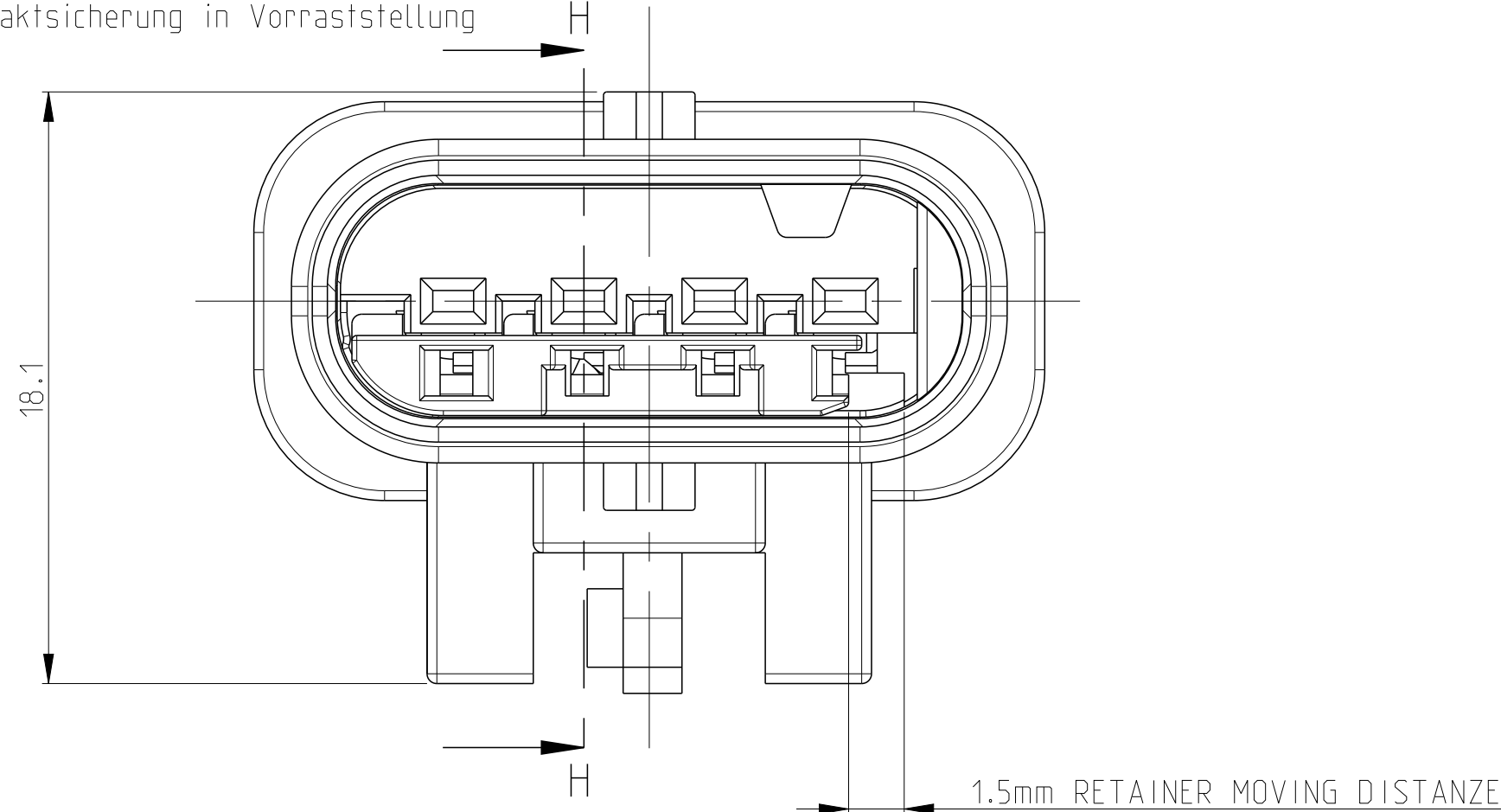
RETAINER IN PRE LOCKED POSITION Kontaktsicherung in Vorraststellung
