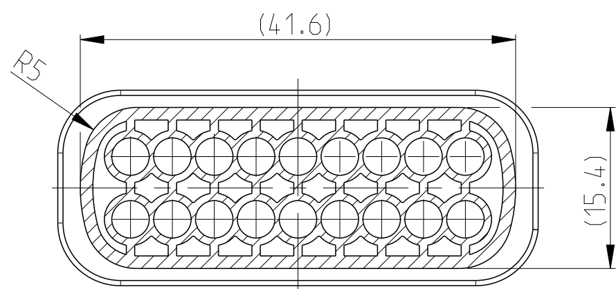
SECTION H-H Schnitt
