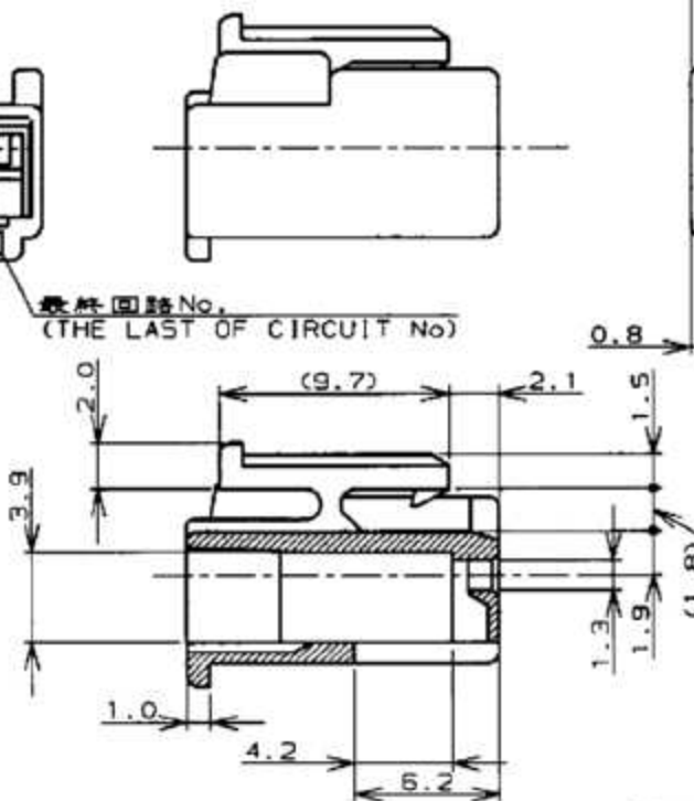
断面 A SECT A
