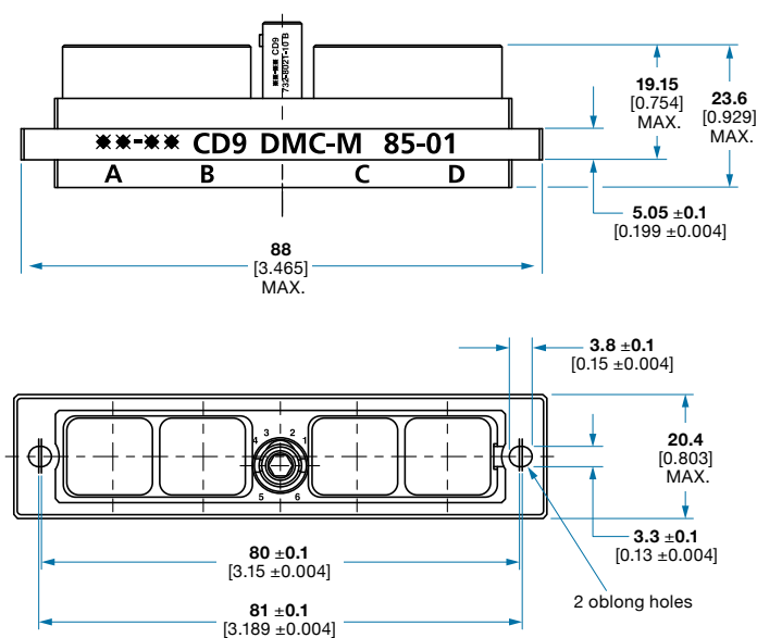
DMC-M 85-01: 4 Modules
