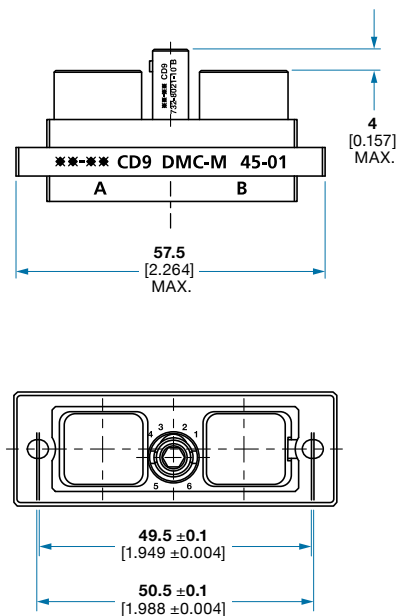
DMC-M 45-01: 2 Modules
