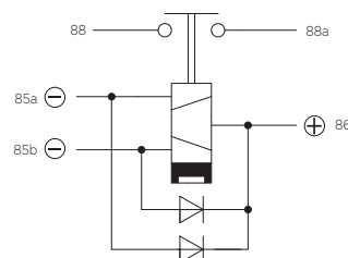
Suppression diode 30-100-59
