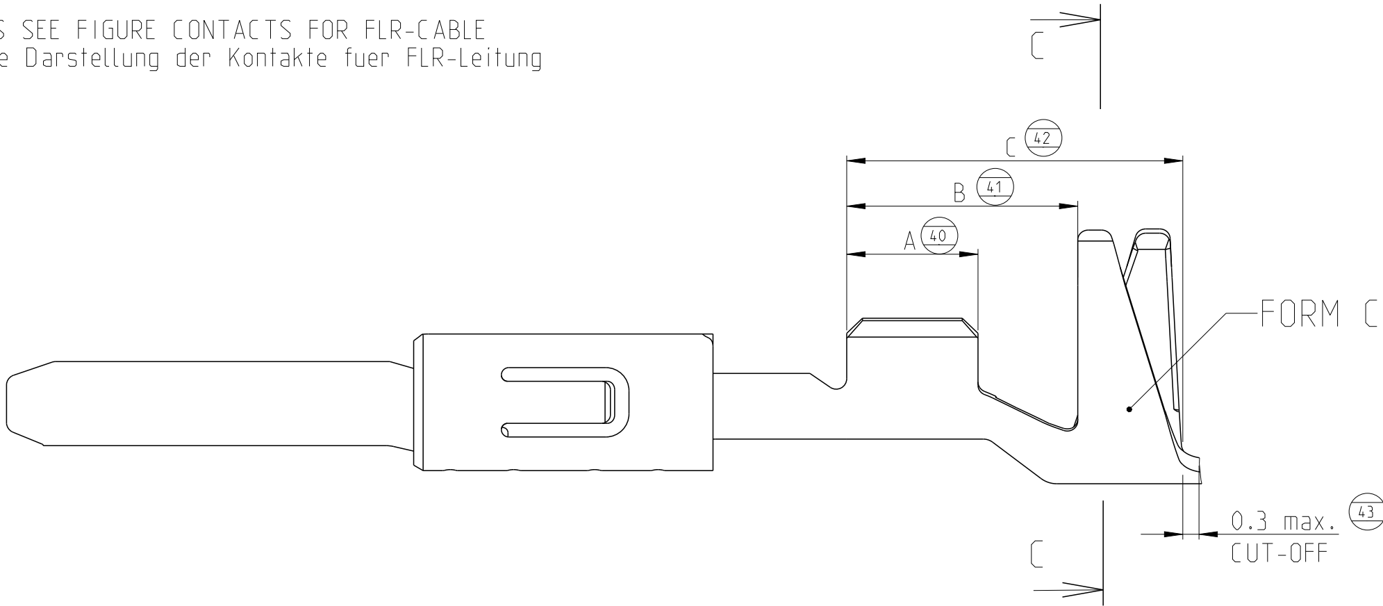
CONTACTS FOR SINGLE WIRE SEALING SYSTEM: FLR- AND FLK-CABLE Kontakte fuer Einzeldichtung-System: FLR- und FLK-Leitung
