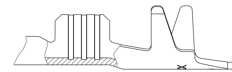
DESIGN 2 Ausfuehrung 2
