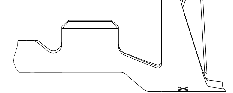
DESIGN 7 Ausfuehrung 7
