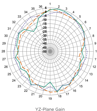
YZ-Plane Gain
