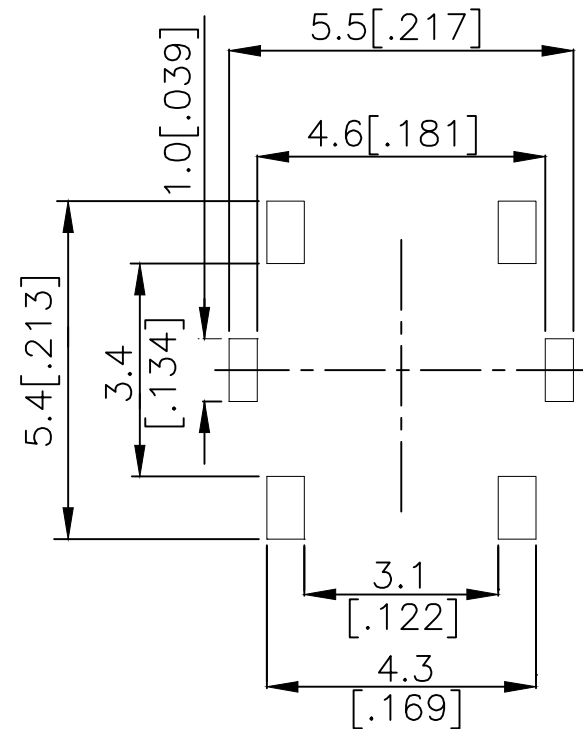
P.C.B. LAYOUT
