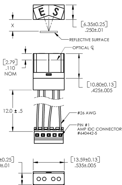
OPB755NZ
