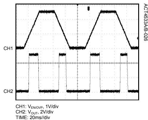
EN/OVP Test
