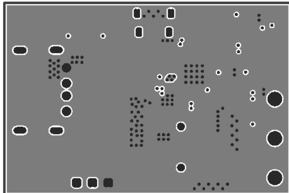
Middle 1 Layer
