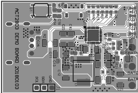
Top Layer
