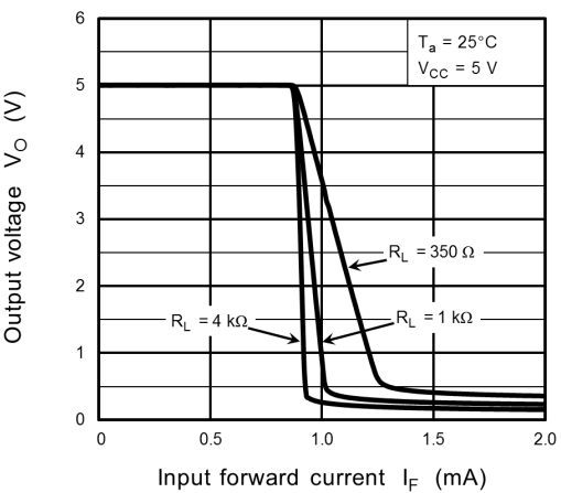
Fig. 11.2.8 V_O - I_F
