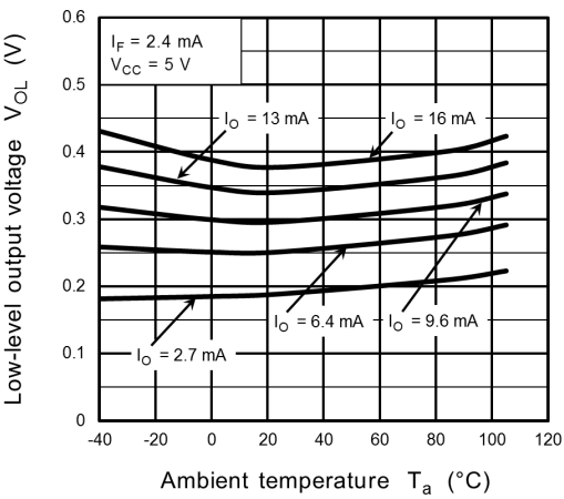
Fig. 11.2.4 V_{OL} - T_a
