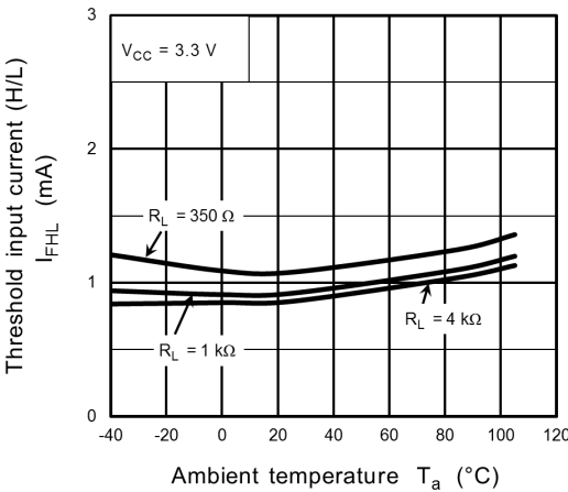
Fig. 11.2.9 I_{FHL} - T_a
