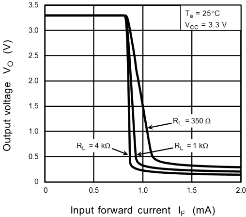
Fig. 11.2.7 V_O - I_F
