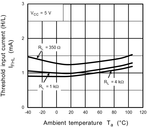
Fig. 11.2.10 I_{FHL} - T_a
