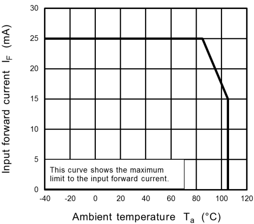
Fig. 11.2.2 I_F - T_a
