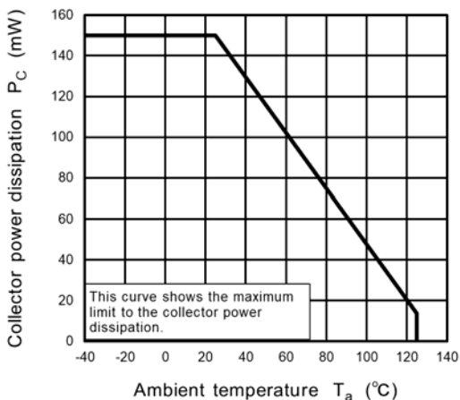
Fig. 12.2 P_C - T_a
