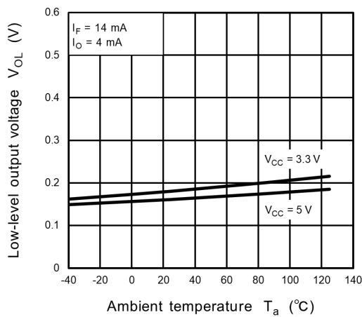
Fig. 14.2.3 V_{OL} - T_a
