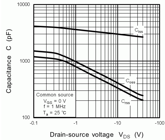
Fig. 8.13 Capacitance - V_{DS}
