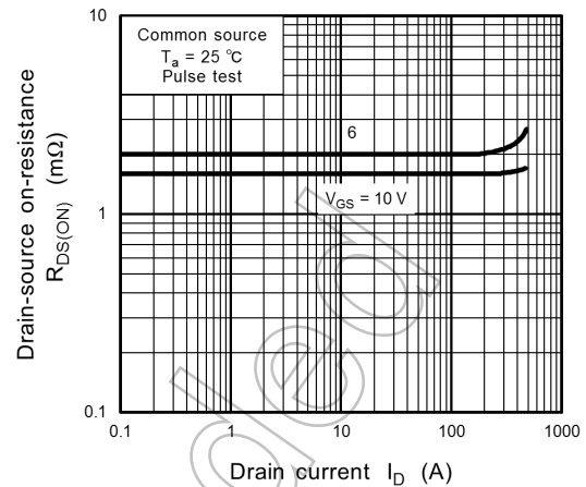
Fig. 9.8 R_{DS(ON)} - I_D
