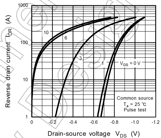
Fig. 9.10 I_{DR} - V_{DS}
