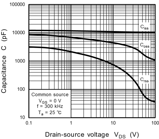
Fig. 9.13 Capacitance - V_{DS}
