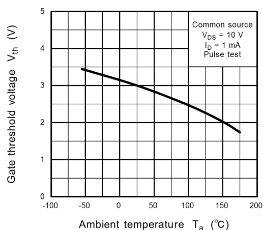
Fig. 9.12 V_{th} - T_a
