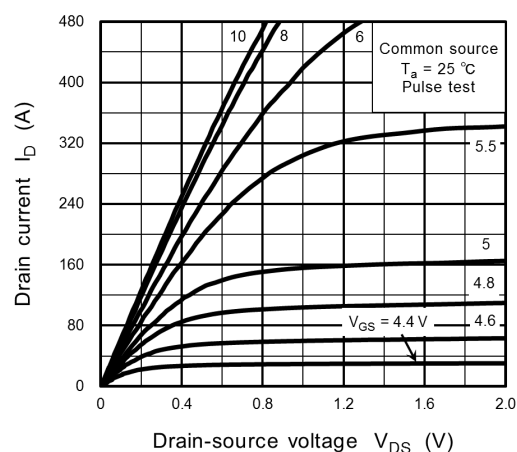
Fig. 9.2 I_D - V_{DS}
