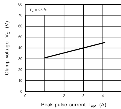
Fig. 10.18.2 V_C - I_{PP}
