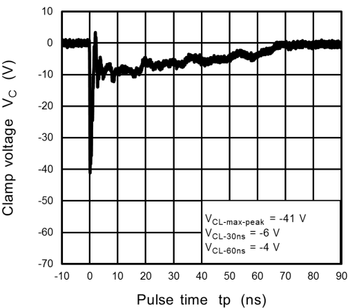
Fig. 6.1.2 -8 kV
