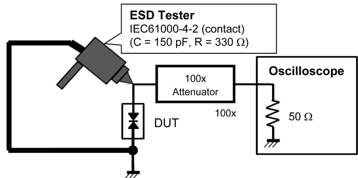
Fig. 6.1.3 IEC61000-4-2 (Contact)
