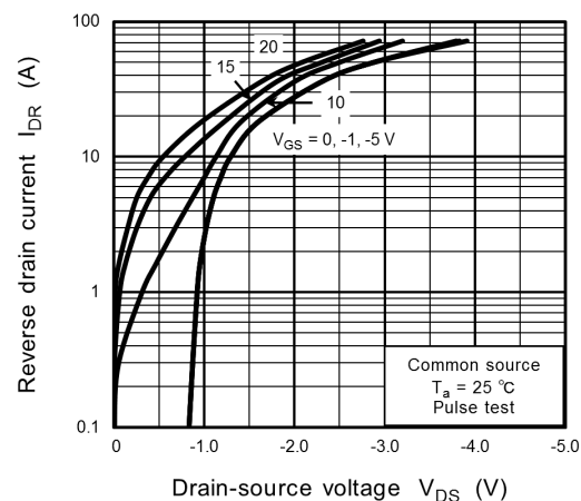
Fig. 8.14 I_{DR} - V_{DS}
