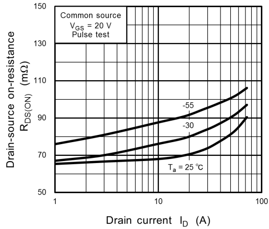
Fig. 8.7 R_{DS(ON)} - I_D
