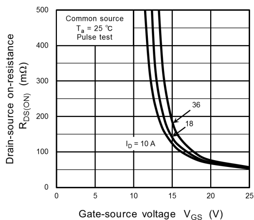
Fig. 8.5 R_{DS(ON)} - V_{GS}
