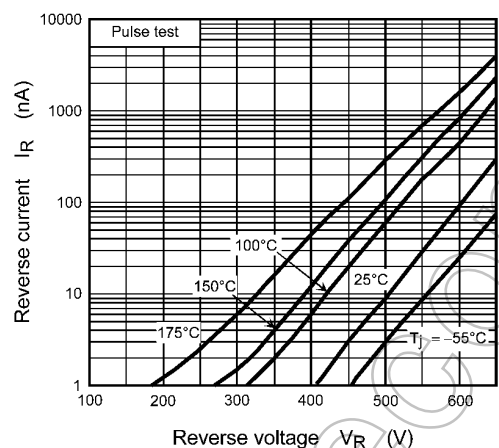
Fig. 9.3 I_R - V_R
