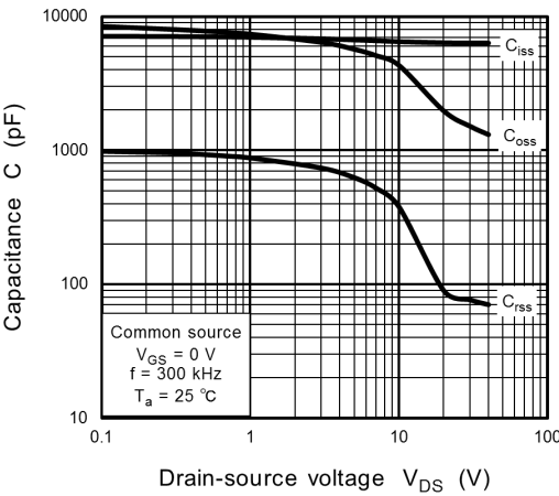
Fig. 8.13 Capacitance - V_{DS}
