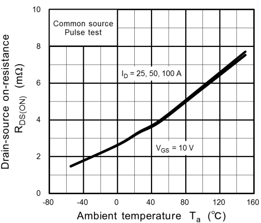
Fig. 8.9 R_{DS(ON)} - T_a
