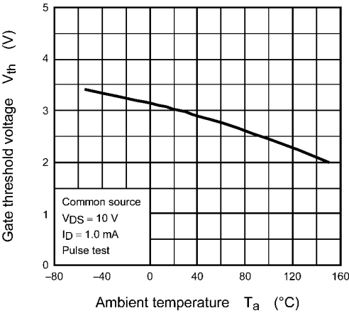
Fig. 8.9 V_{th} - T_a
