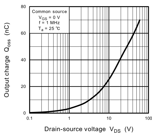
Fig. 8.12 Q_{oss} - V_{DS}
