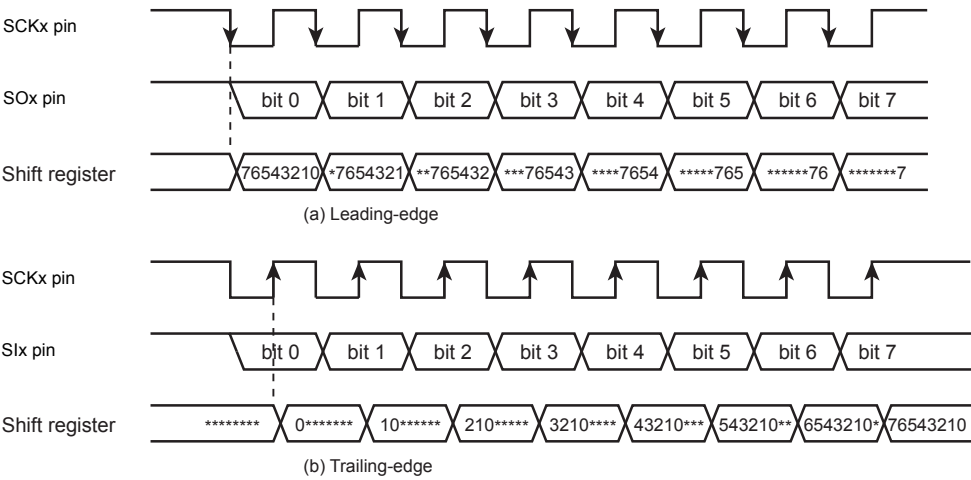
Figure 14-17 Shift Edge
