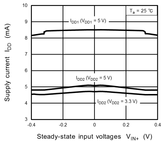
Fig. 12.6 I_{DD} - V_{IN+}
