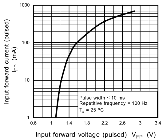
Fig. 12.6 I_{FP} - V_{FP}
