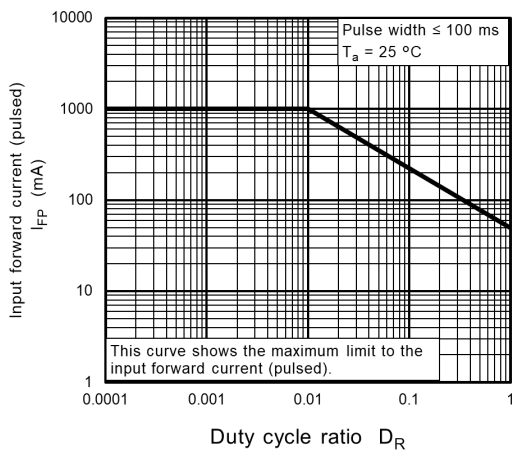
Fig. 12.3 I_{FP} - D_R
