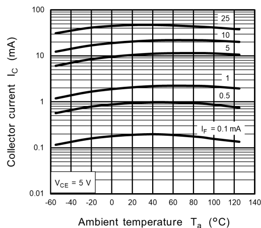
Fig. 12.13 I_C - T_a
