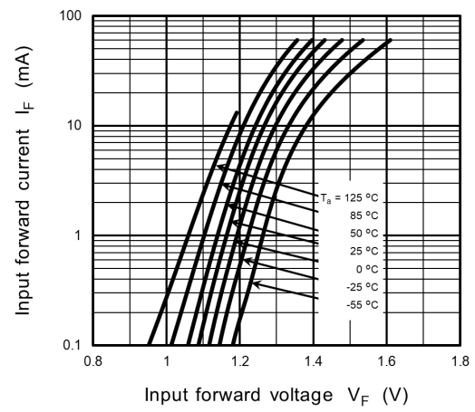
Fig. 12.4 I_F - V_F
