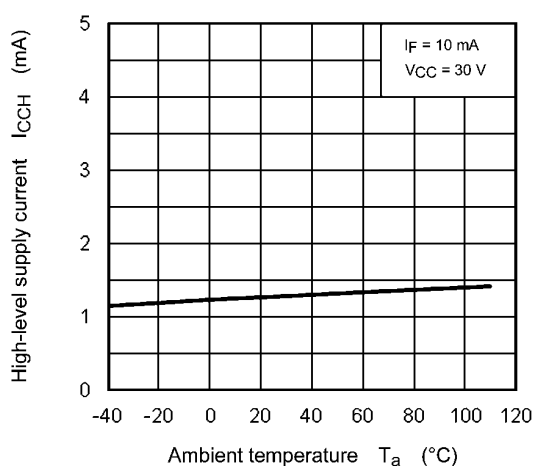
Fig. 12.2.6 I_{CCH} - T_a
