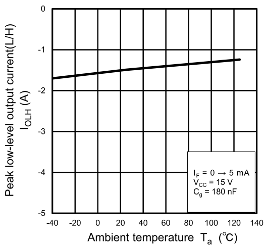
Fig. 13.2.11 I_{OLH} - T_a
