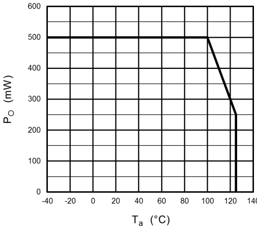
Fig. 13.2.3 P_O - T_a
