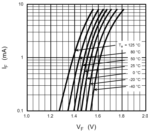
Fig. 13.2.1 I_F - V_F
