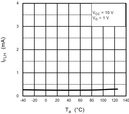
Fig. 13.2.4 I_{FLH} - T_a
