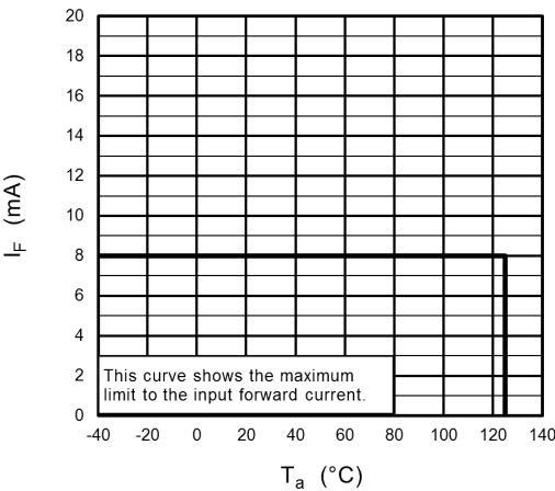
Fig. 13.2.2 I_F - T_a
