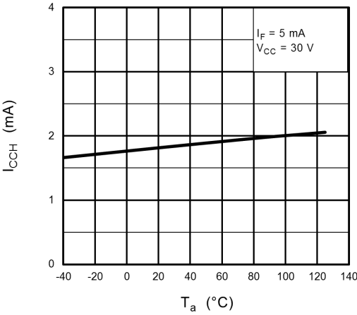
Fig. 13.2.6 I_{CCH} - T_a
