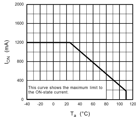
Fig. 14.2 I_{\text{ON}} - T_a
