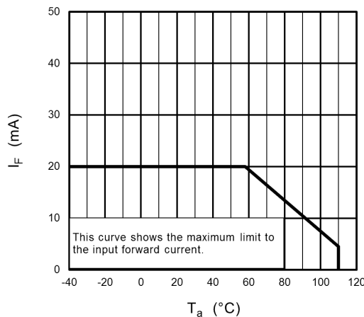
Fig. 14.1 I_F - T_a
