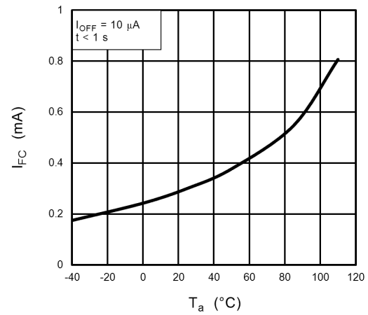
Fig. 14.6 I_{FC} - T_a
