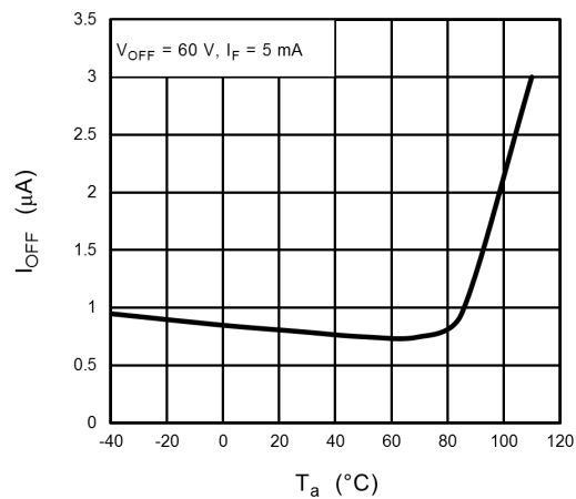
Fig. 14.9 I_{OFF} - T_a
