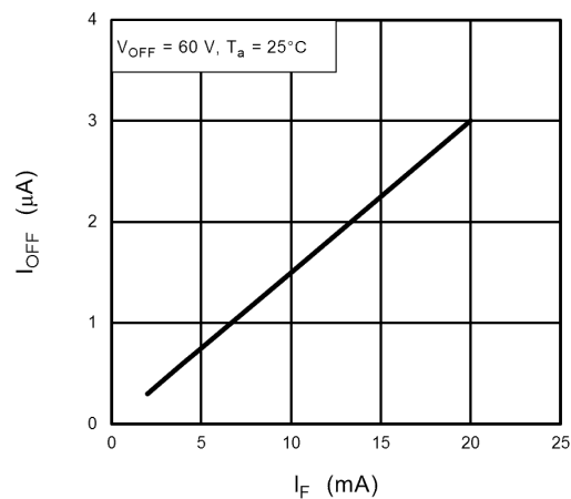
Fig. 14.11 I_{OFF} - I_F
