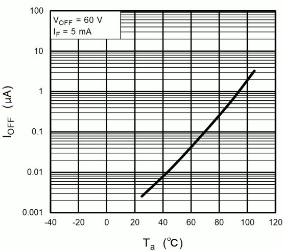
Fig. 12.8 I_{OFF} - T_a
