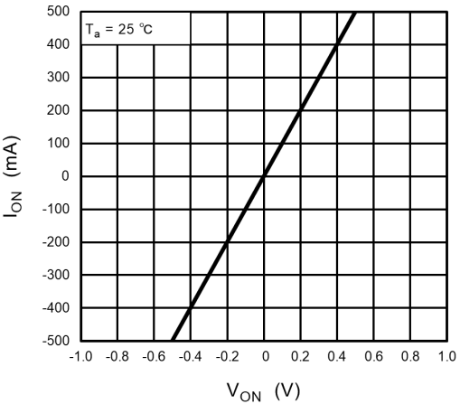
Fig. 12.4 I_{ON} - V_{ON}
