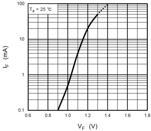
Fig. 12.3 I_F - V_F
