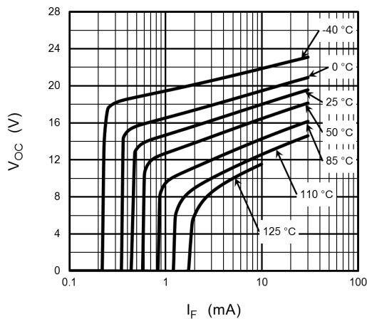
Fig. 12.5 V_{OC} - I_F
