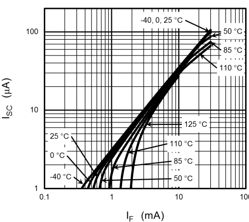
Fig. 12.6 I_{SC} - I_F
