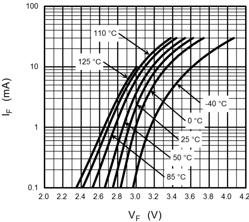
Fig. 12.2 I_F - V_F
