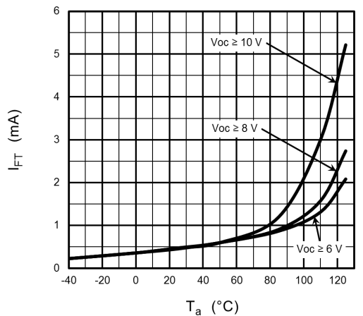
Fig. 12.3 I_{FT} - T_a
