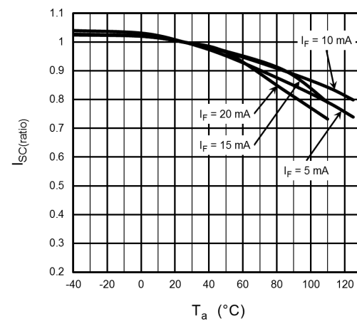
Fig. 12.10 I_{SC(ratio)} - T_a
