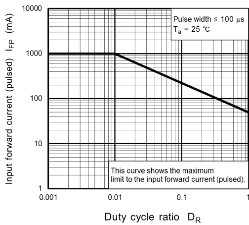
Fig. 11.3 I_{FP} - D_R
