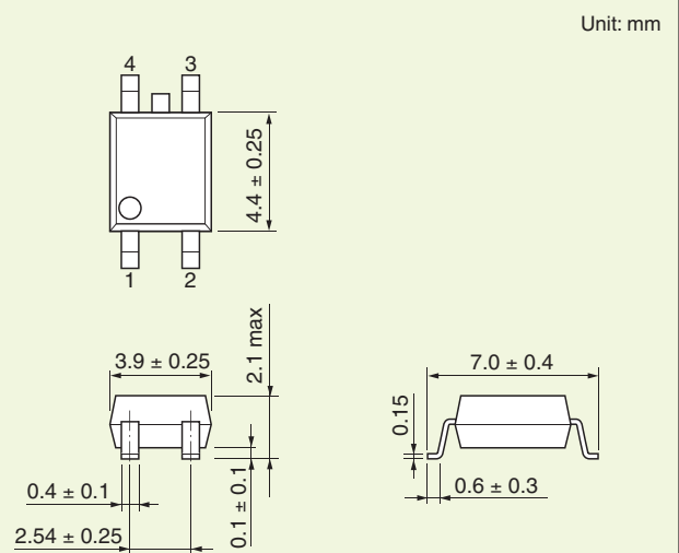
2.54SOP4
