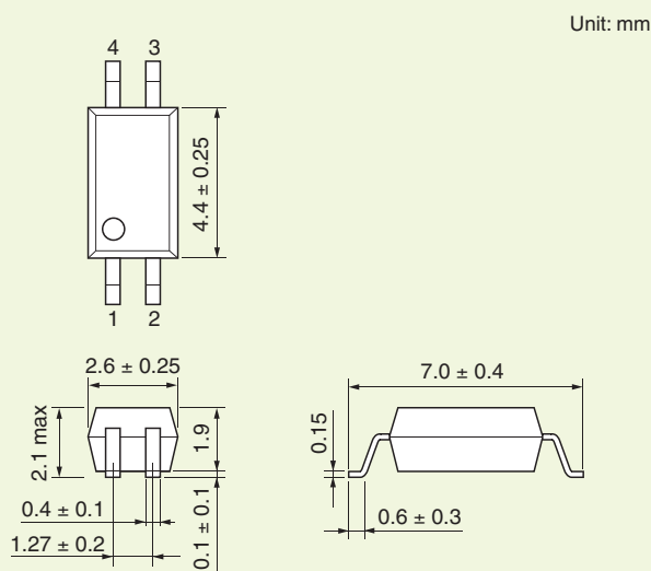
SOP4
