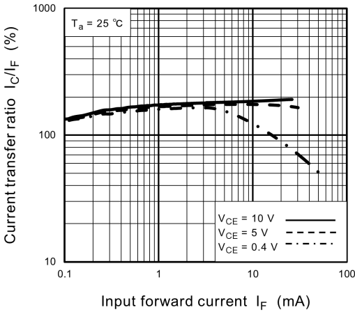
Fig. 11.12 I_C/I_F - I_F
