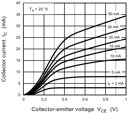
Fig. 11.8 I_C - V_{CE}
