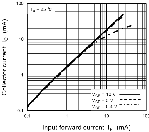
Fig. 11.11 I_C - I_F
