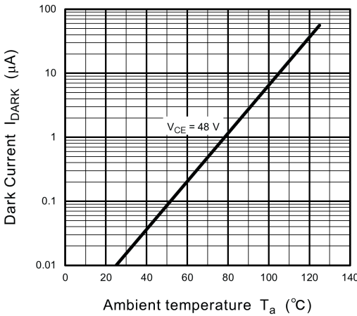
Fig. 11.9 I_{DARK} - T_a
