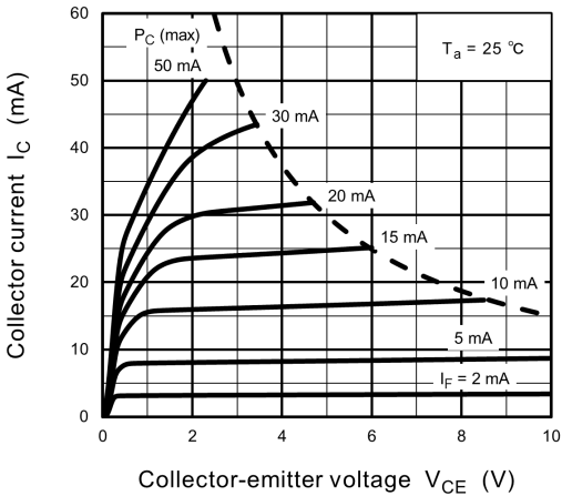
Fig. 11.7 I_C - V_{CE}
