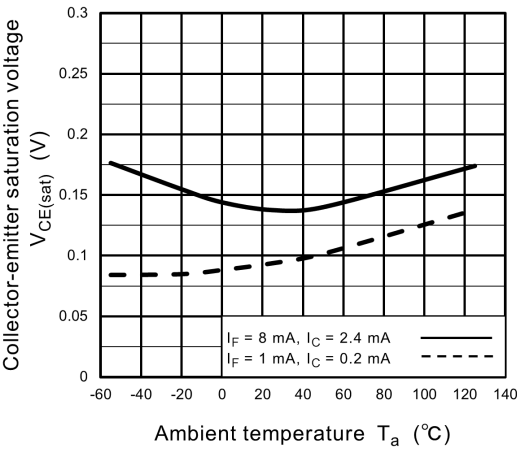
Fig. 11.10 V_{CE(sat)} - T_a
