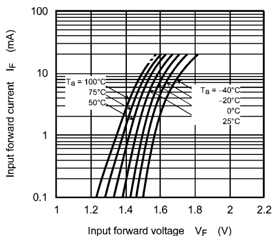
Fig. 12.2.1 I_F - V_F
