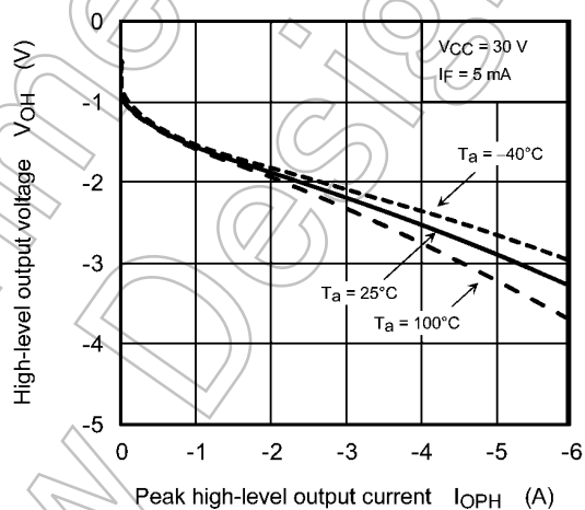
Fig. 12.2.10 V_{OH} - I_{OPH}
