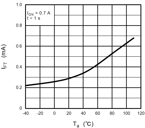
Fig. 16.1.6 I_{FT} - T_a
