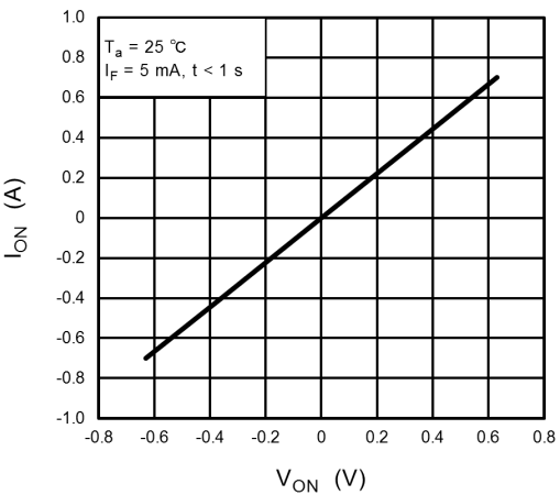
Fig. 16.1.4 I_{ON} - V_{ON}
