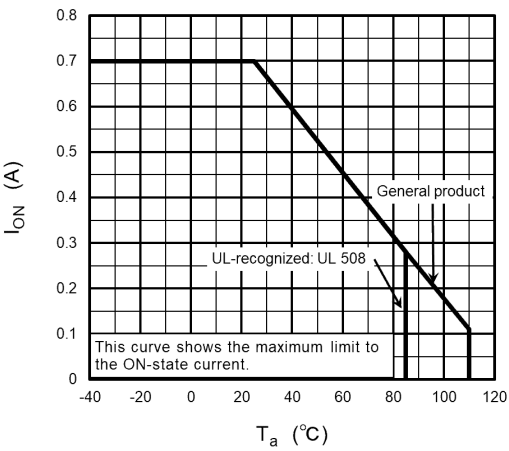
Fig. 16.1.2 I_{ON} - T_a
